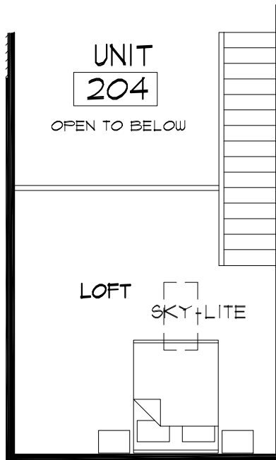
LOFT PLAN
